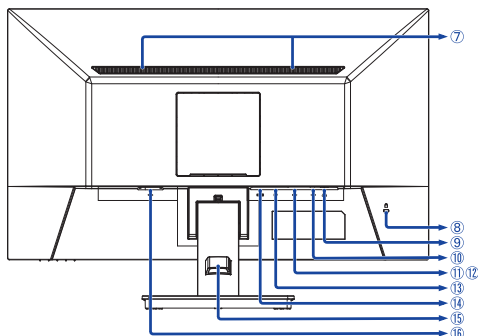
<Zadní>
